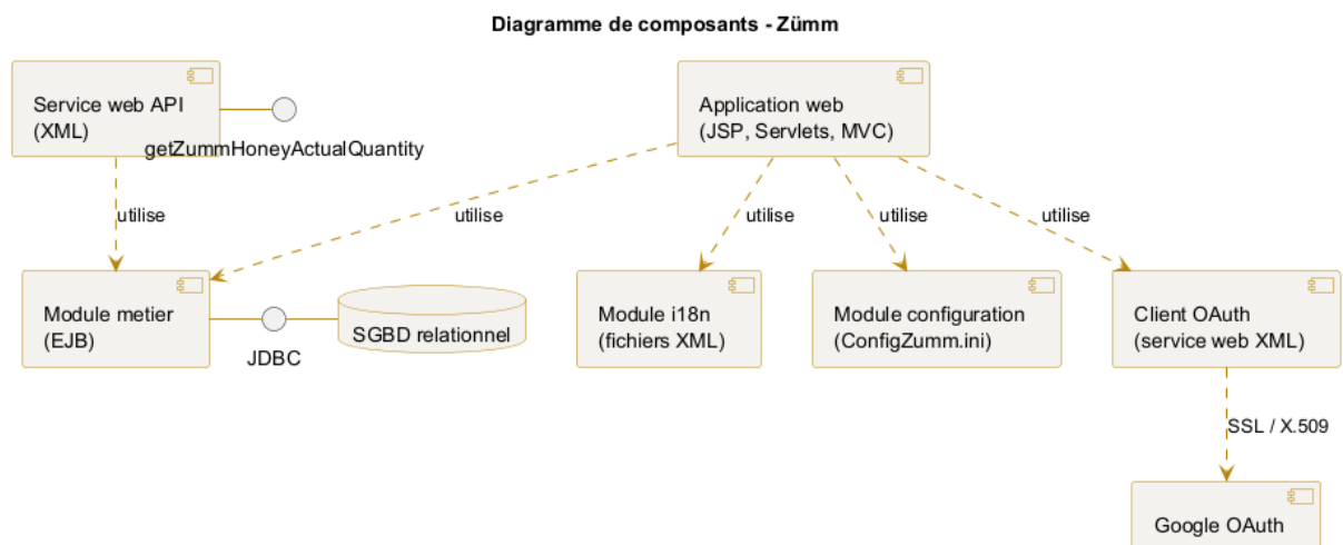
Figure 7.10. Diagramme de composants du système Zümm.
